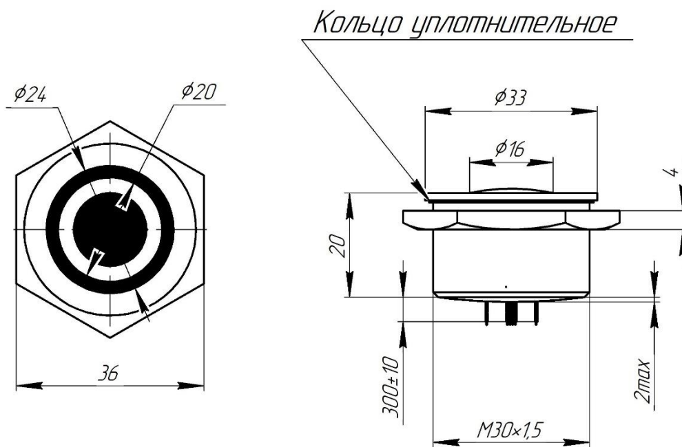
Рисунок 3 – Габаритные размеры изделия
